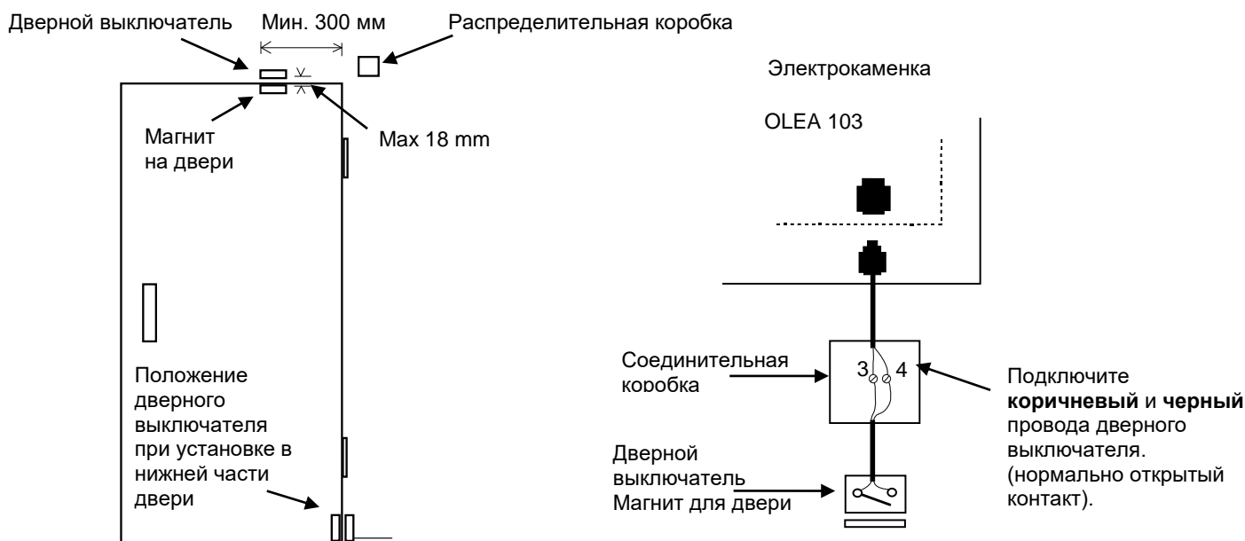
Рис. 5. Установка дверного выключателя
