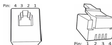
Рис 6. Расположение выводов разъема RJ10 печатной платы.
