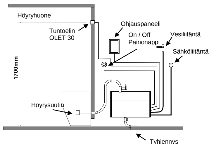
Ohjauspaneelin sijoitus
