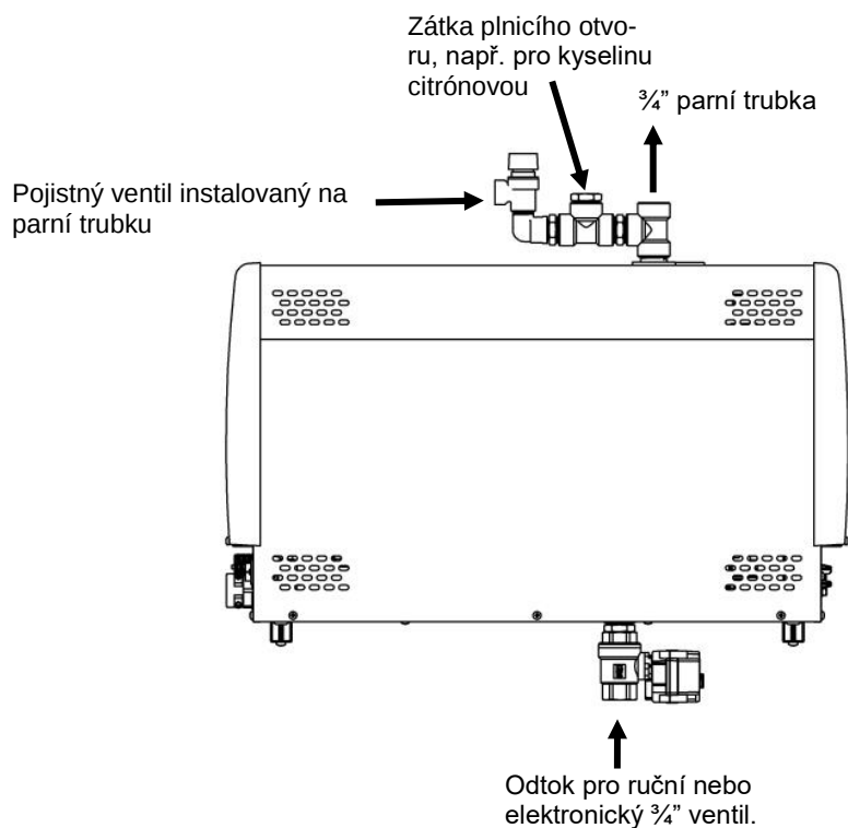
Obrázek. Instalace pojistného ventilu a automatického vypouštěcího ventilu (Příslušenství automatic drain valve). Viz schéma obvodu zapojení.
