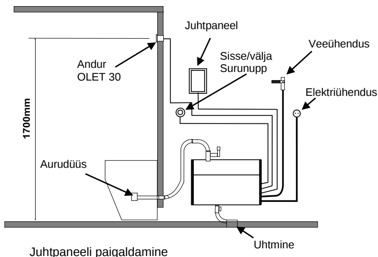
Juhtpaneeli paigaldamine
