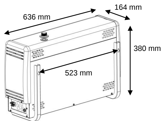
Aurugeneraatori seinalle paigaldamine
