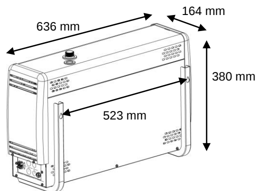
A gőzfejlesztő felszerelése a falra
