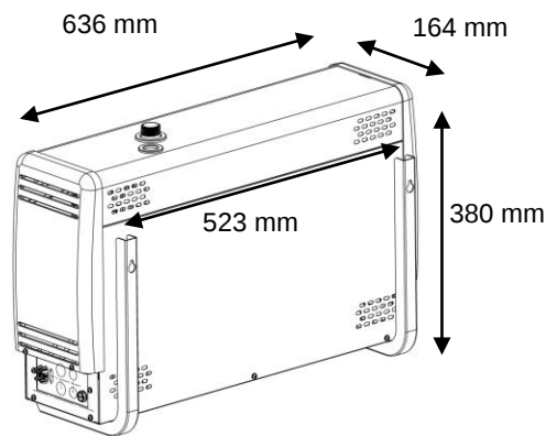
Hörygeneraattorin seinäkiinnitys
